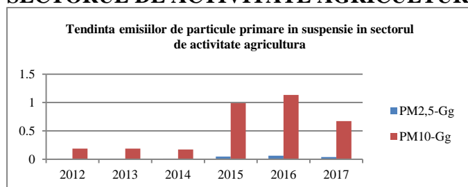
Figura nr. 3-31 Tendința emisiilor de particule primare în suspensie din sectorul de activitate agricolă
