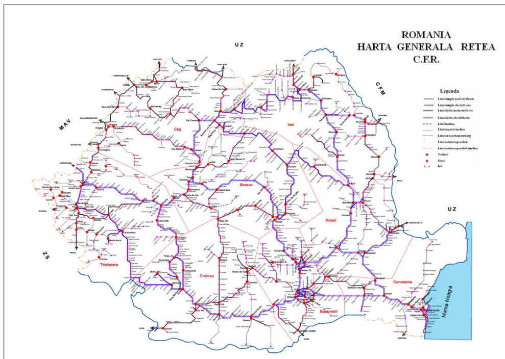
Figura nr. 2-32 Harta Generala Retea CFR
