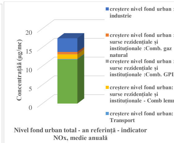
Figura nr. 3-89 Nivel fond urban total – indicator NO x
