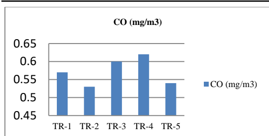
Figura nr. 3-36 Concentrații medii anuale de CO înregistrate la stațiile automate
