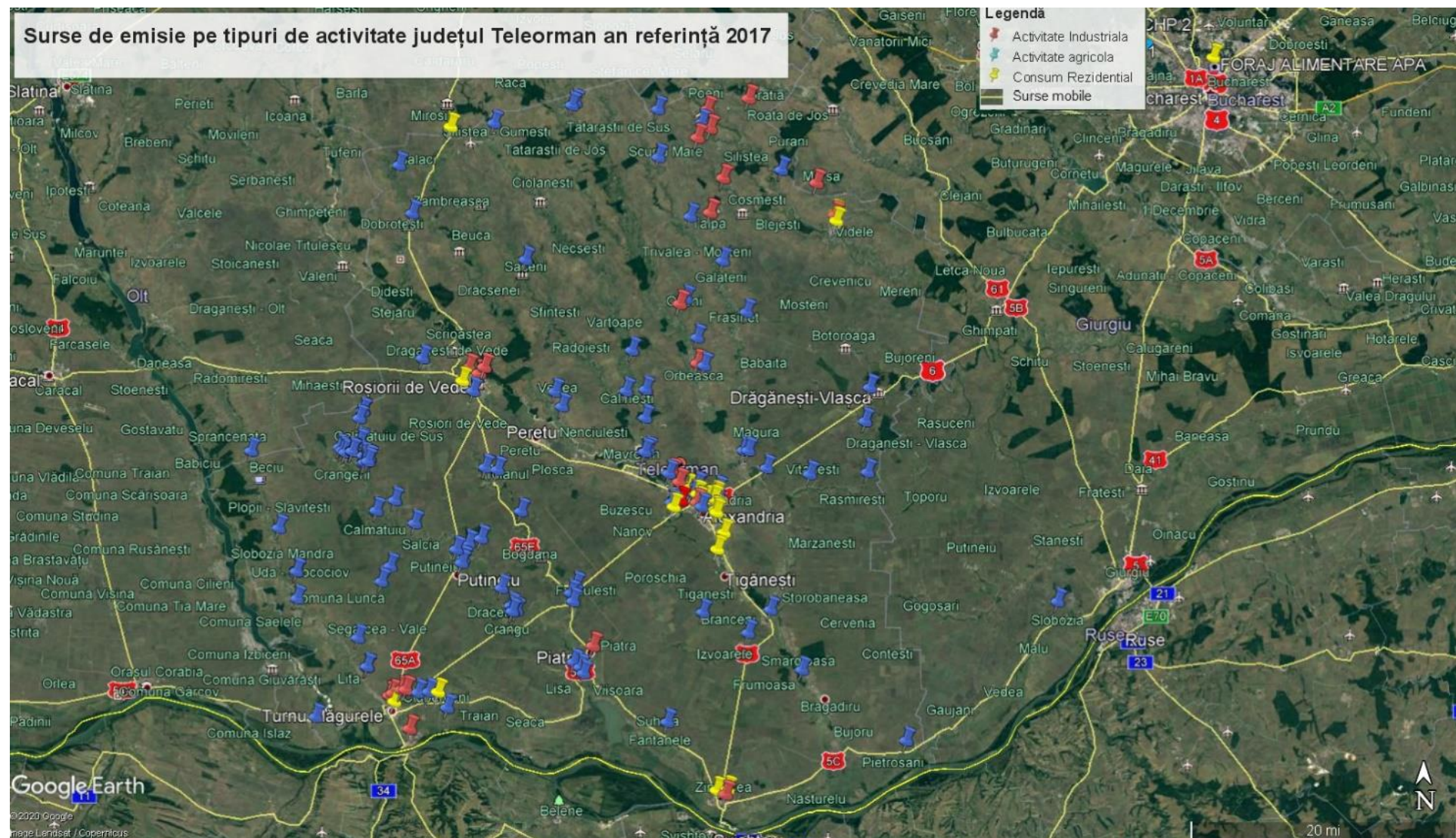
Figura nr. 4-3 Harta surselor de emisie ZONA TELEORMAN pe tipuri de activitate – an referință 2017
