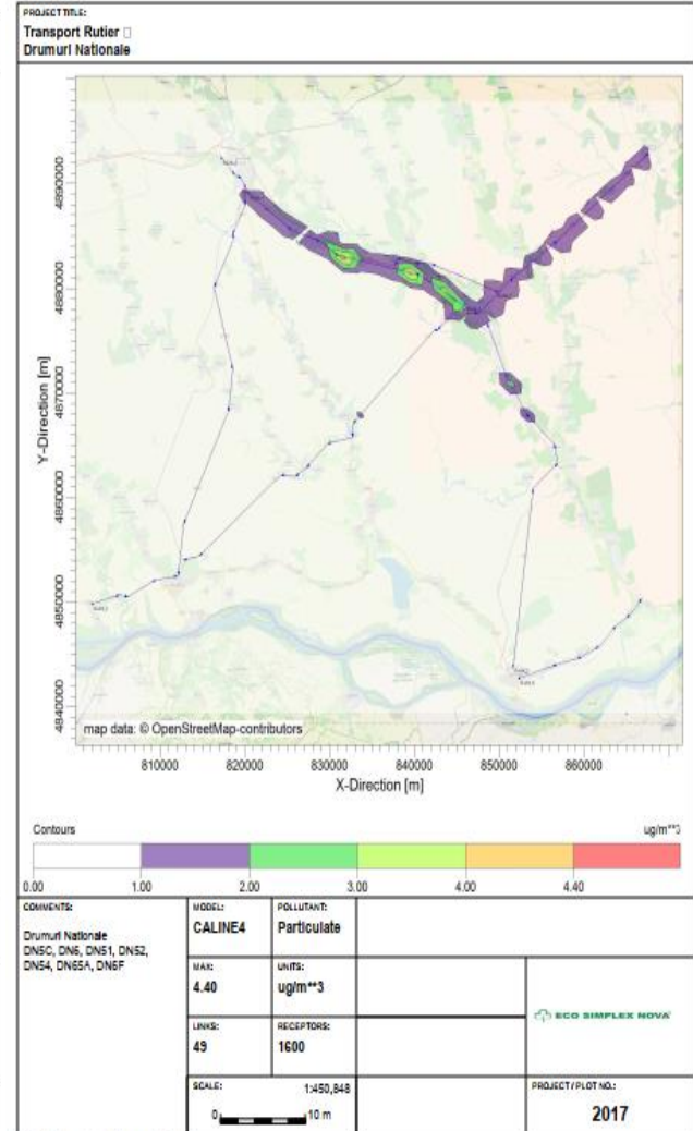
Figura nr. 3-86 Transport rutier – drumuri naționale – indicator PM10
