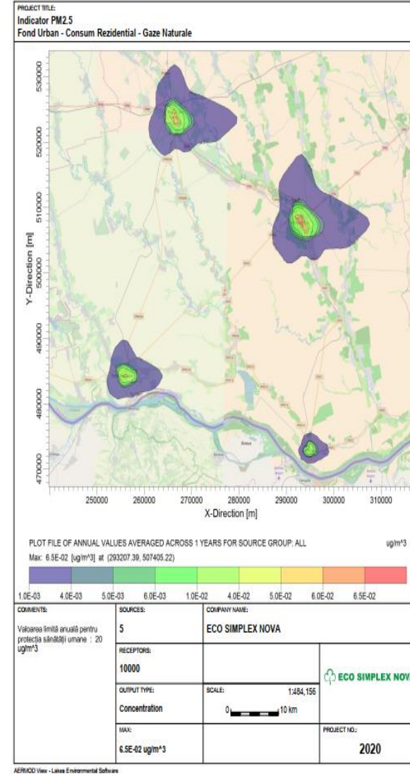
Figura nr. 3-62 Creștere nivel Fond Urban – consum rezidențial GN – indicator PM2,5 medie anuală
