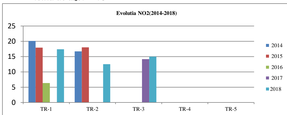
Figura nr. 3-38 Evoluția concentrațiilor medii anuale de NO 2 la stațiile automate
