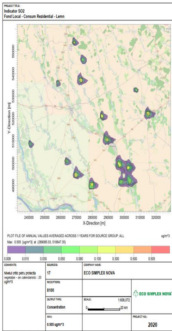
Figura nr. 3-113 Creștere nivel Fond Local — consum rezidențial lemn — indicator SO2, media anuală
