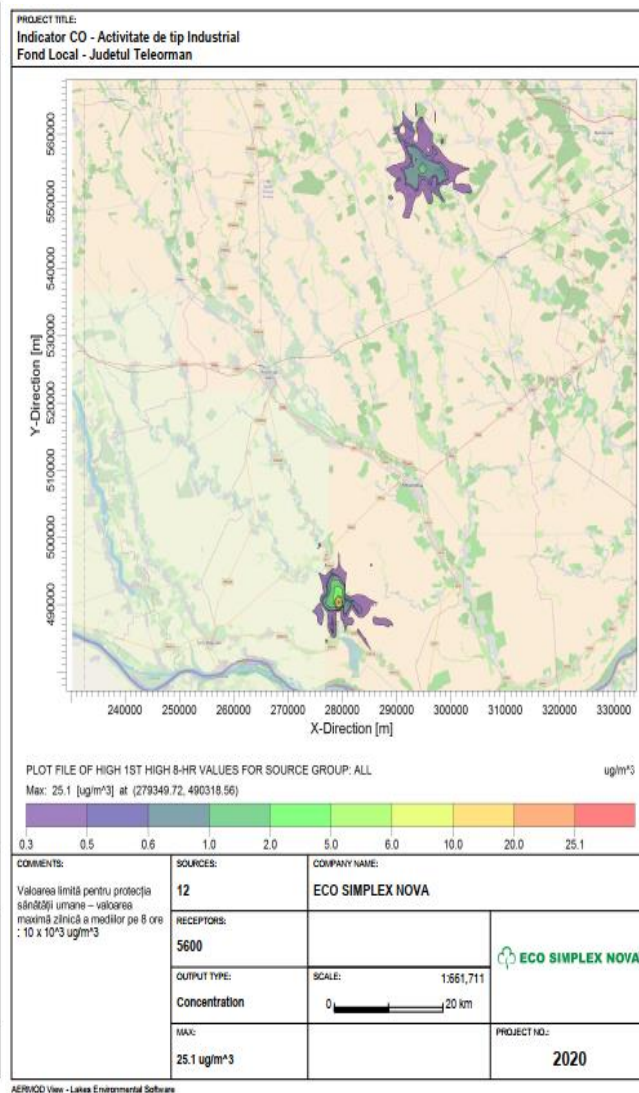
Figura nr. 3-103 Creștere nivel Fond Local –industrie – indicator CO, val max zilnică a mediilor la 8 ore
