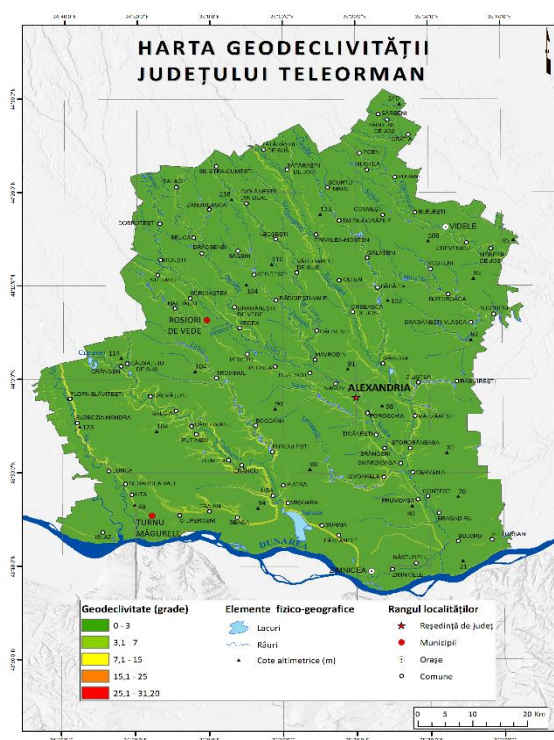
Figura nr. 2-53 Harta geodeclivității județului Teleorman
